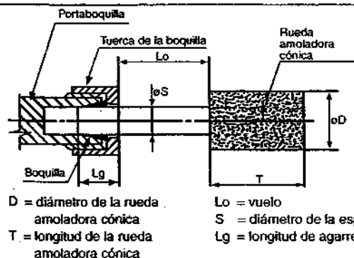
Figura 2. Longitud de agarre de la boquilla y del mandril
