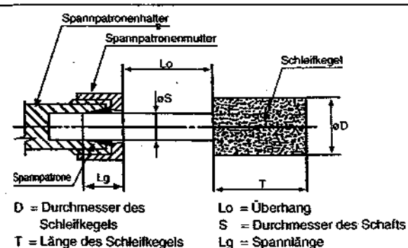
Abbildung 2. Spannlänge der Spannpatrone und des Spannfutters
