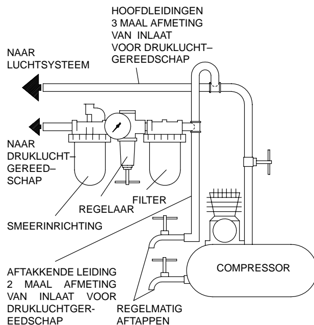
(Tekening TPD905-1)
