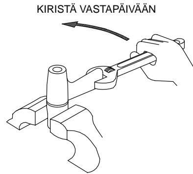
(Kuva TPD1294)
