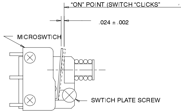
(Dwg. TPD1020)
